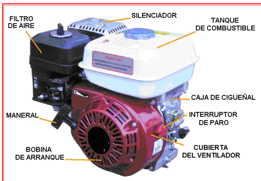
Partes externas del motor de gasolina
